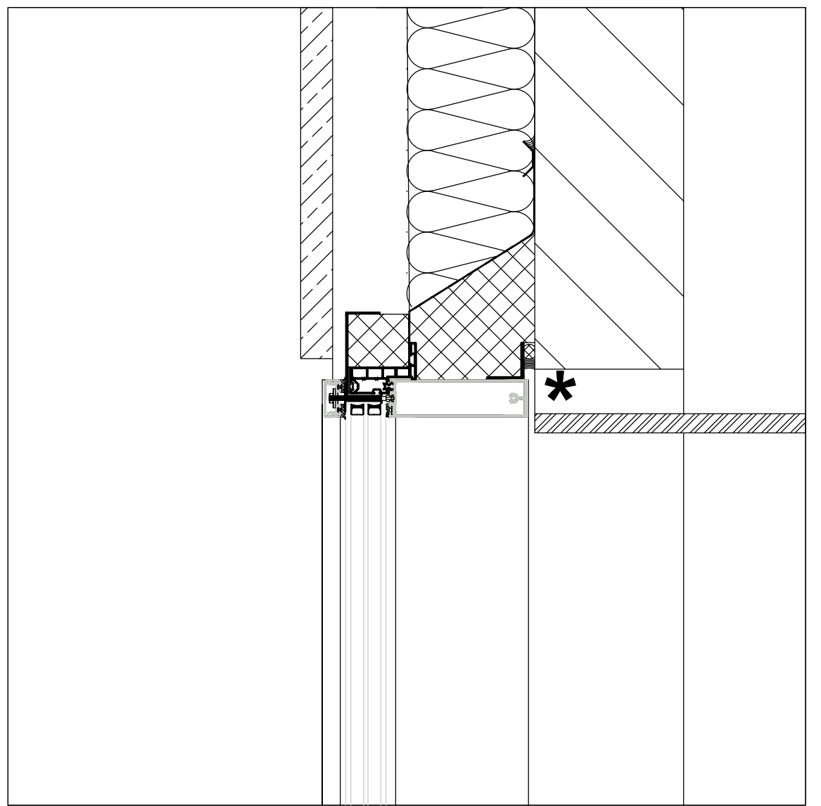
AANSLUITING BOVEN
