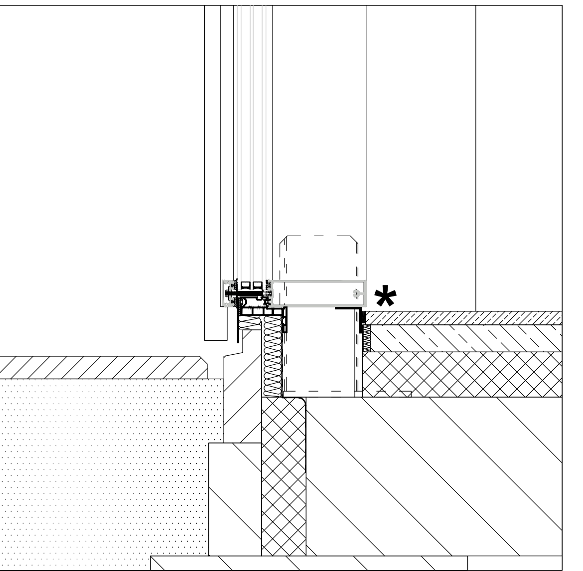
AANSLUITING ONDER
