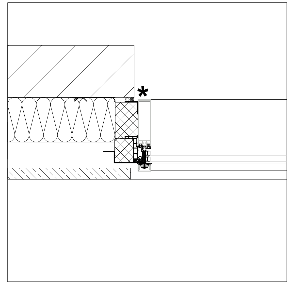
AANSLUITING ZIJ
