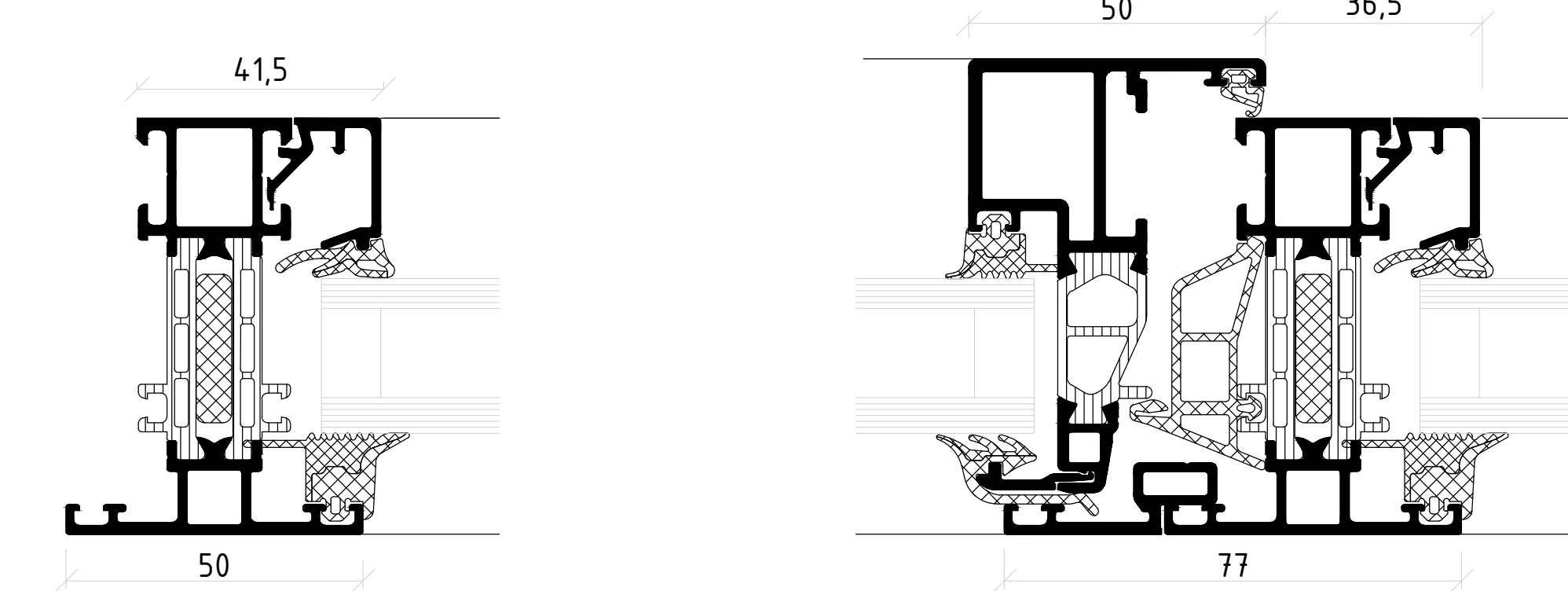
KOZIJN MET VAST GLAS
