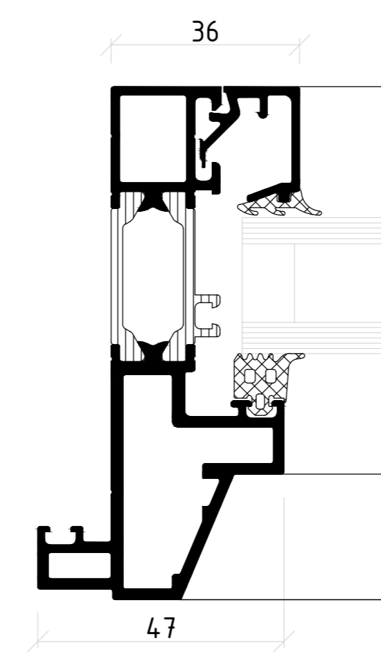
KOZIJN MET VAST GLAS
