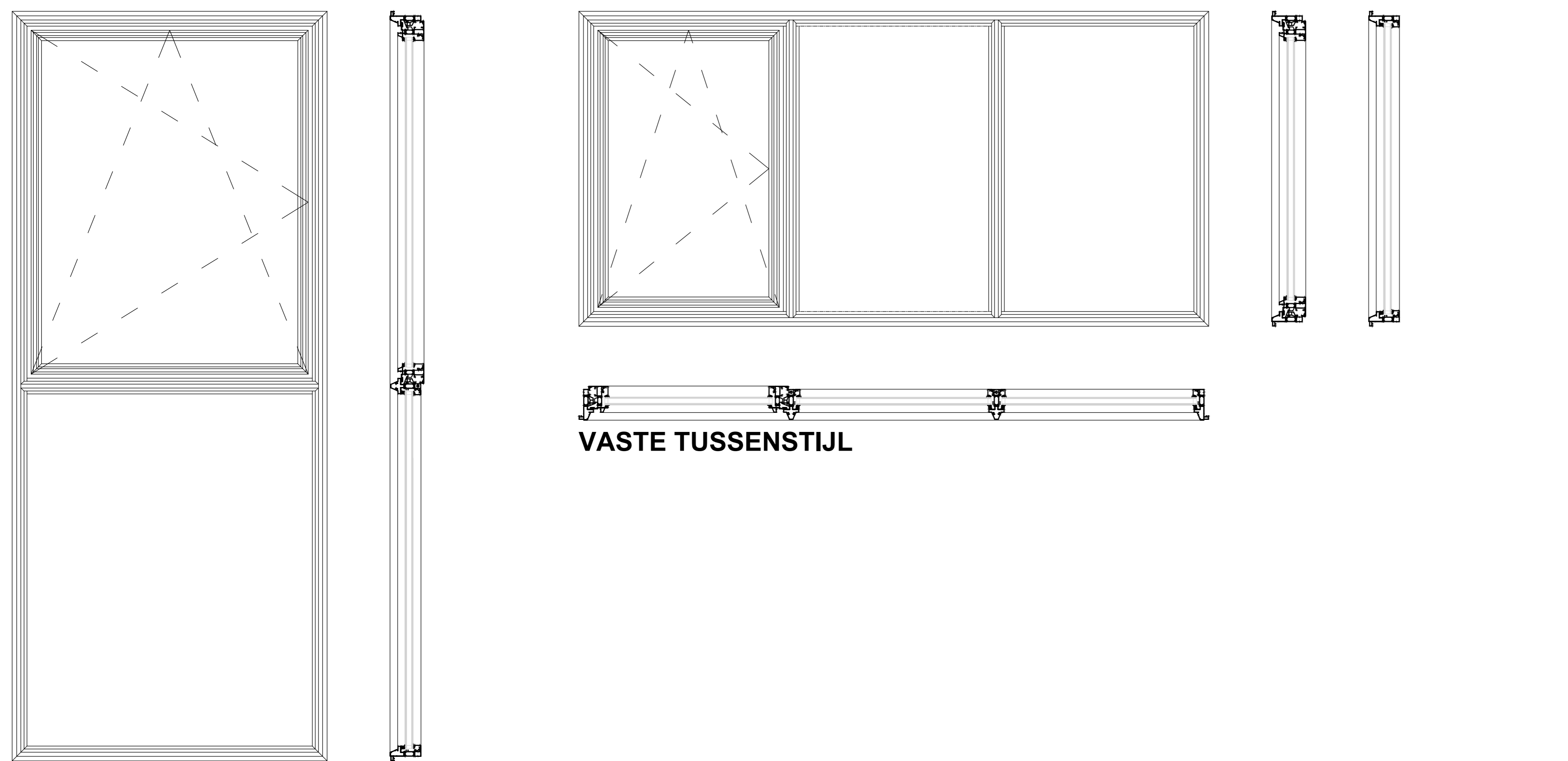
DRAAIKIEPRAAM MET TIP-TRONIC VLEUGEL
