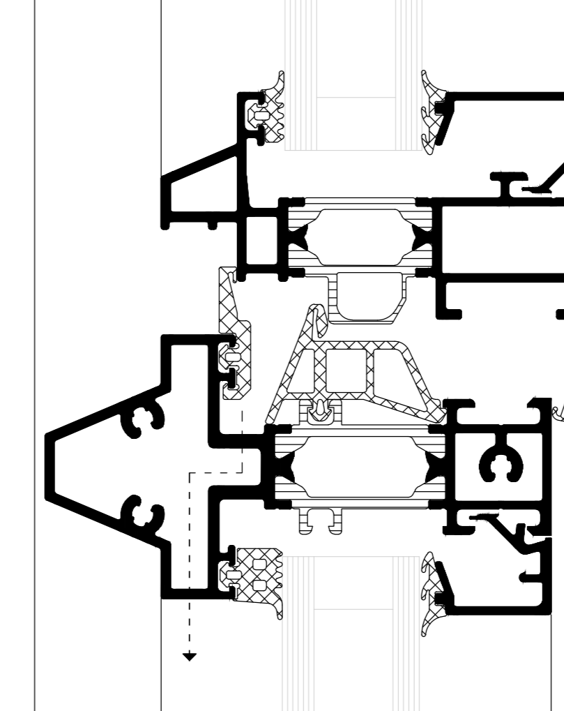
VERBORGEN ONTWATERING BIJ TUSSENREGEL
