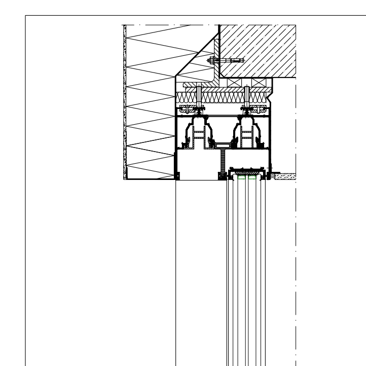
AANSLUITING BOVEN
