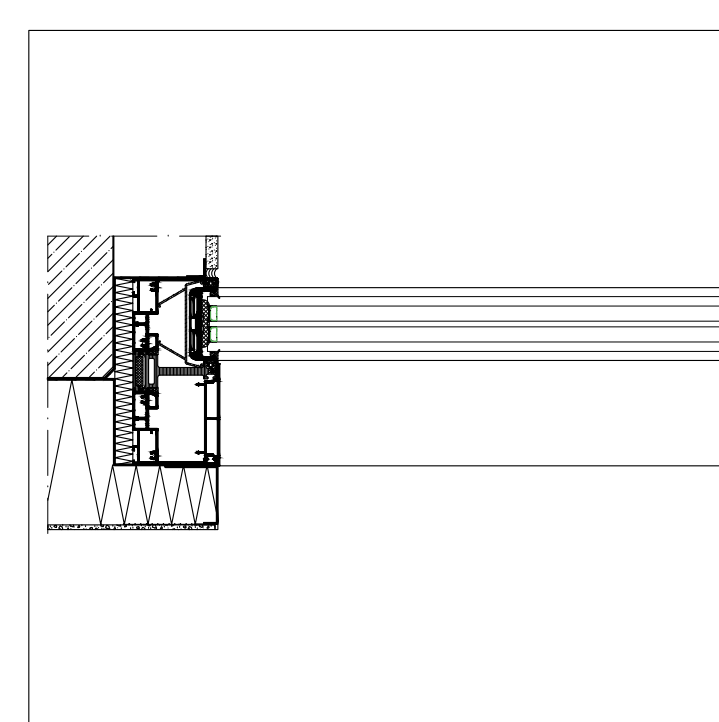
AANSLUITING ZIJ
