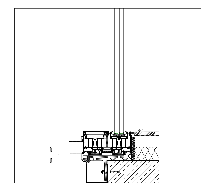
AANSLUITING ONDER
